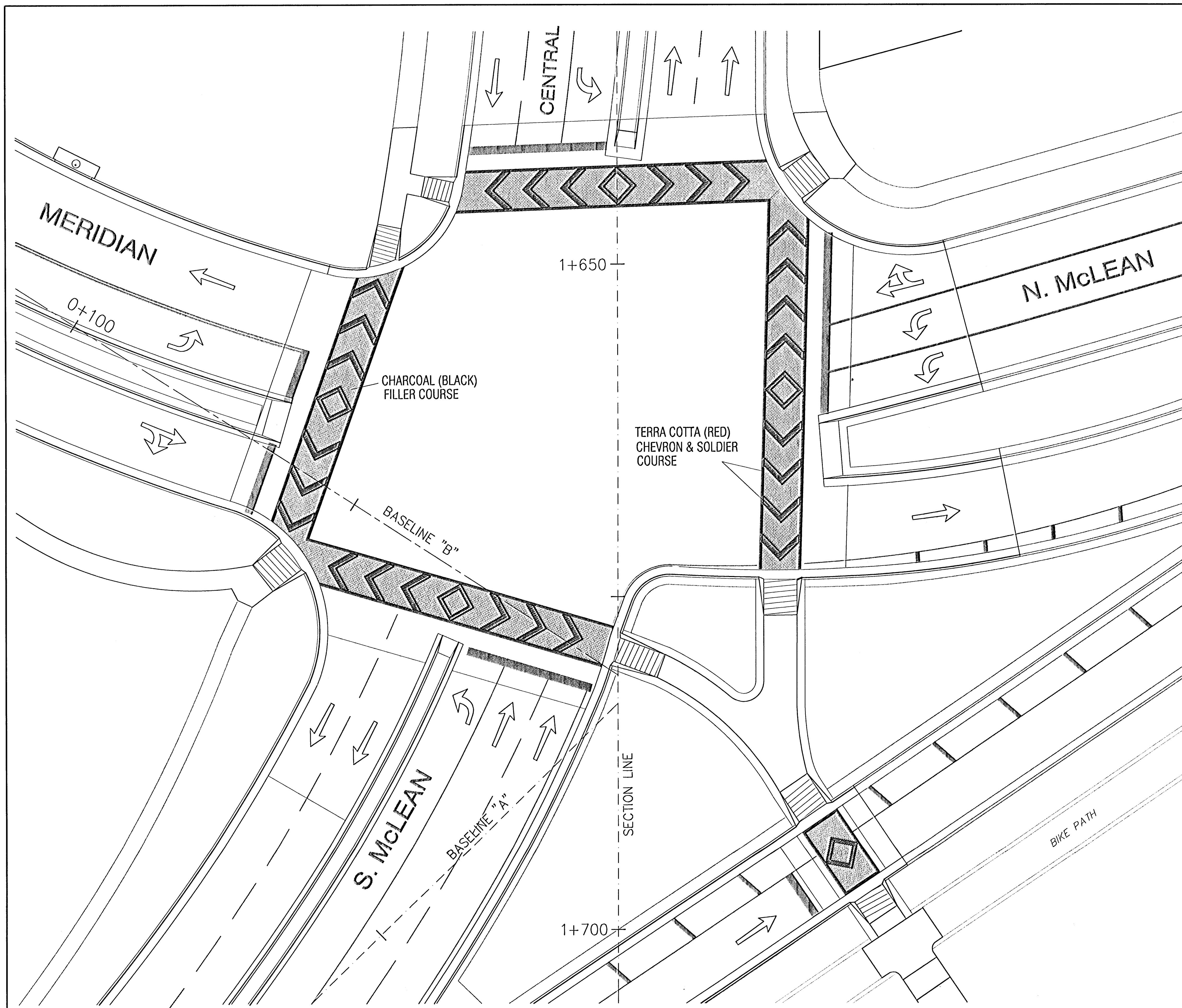
TYPICAL PAVER PATTERNS N.T.S.
