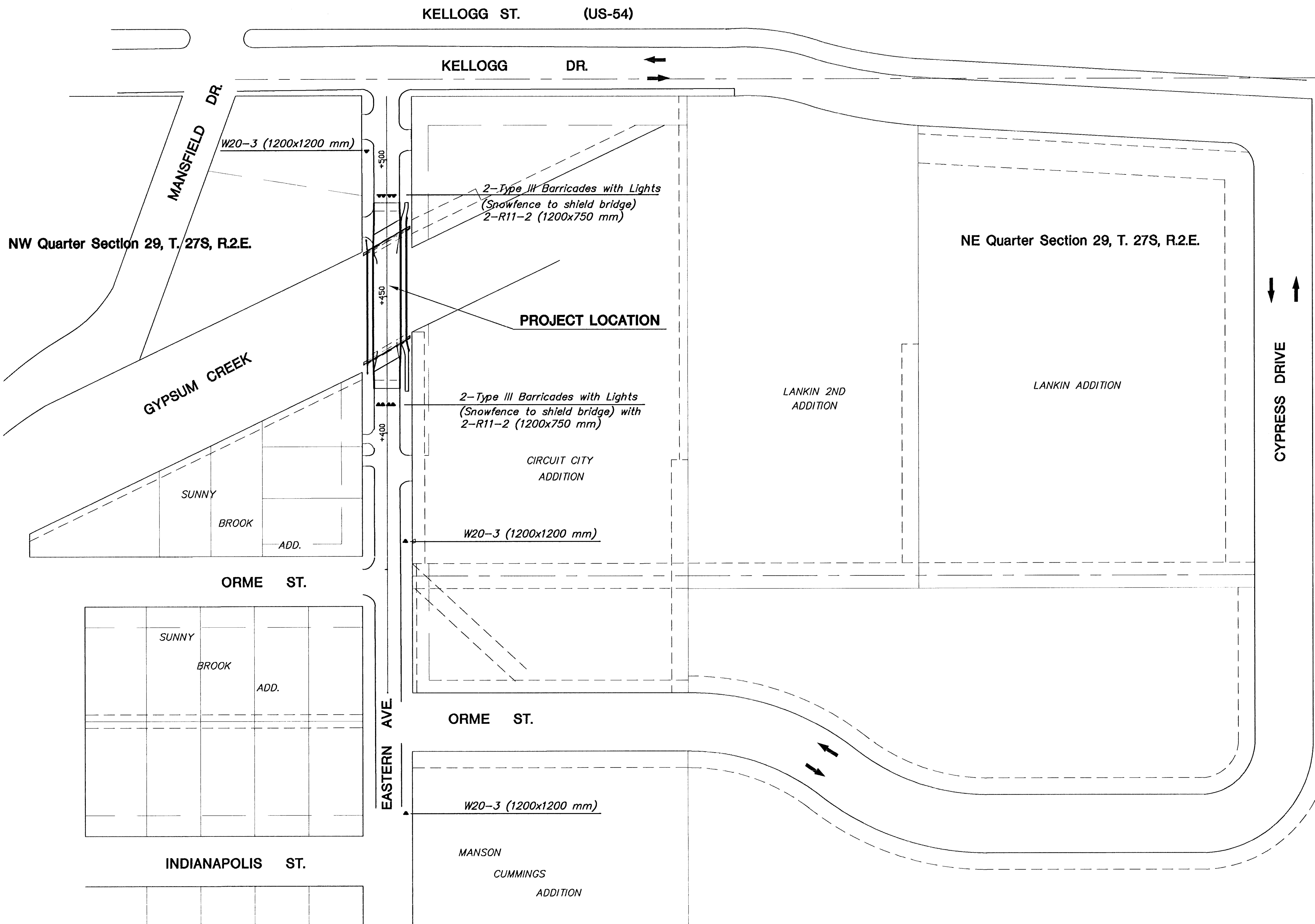
DETOUR PLAN
