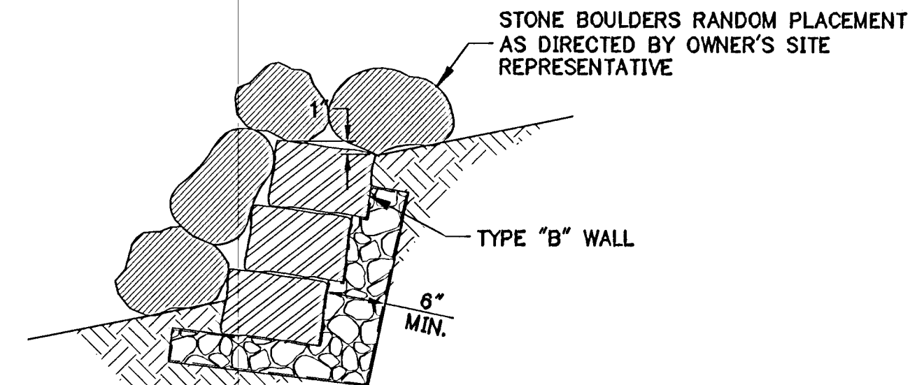
WALL BOULDER SCHEMATIC LAYOUT SCALE: N.T.S.
