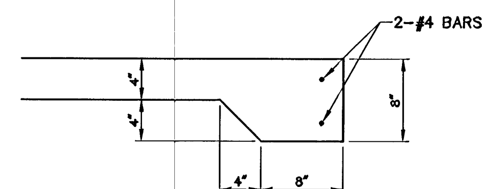
THICKENED EDGE DETAIL SCALE: N.T.S.
