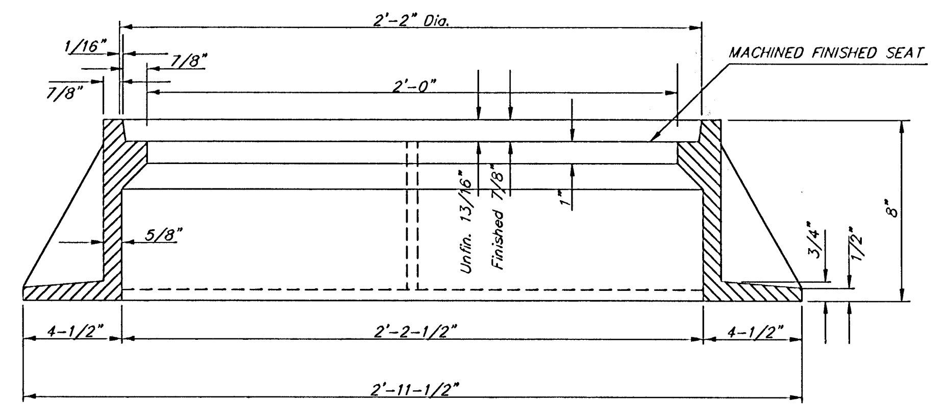
SECTION A-A
