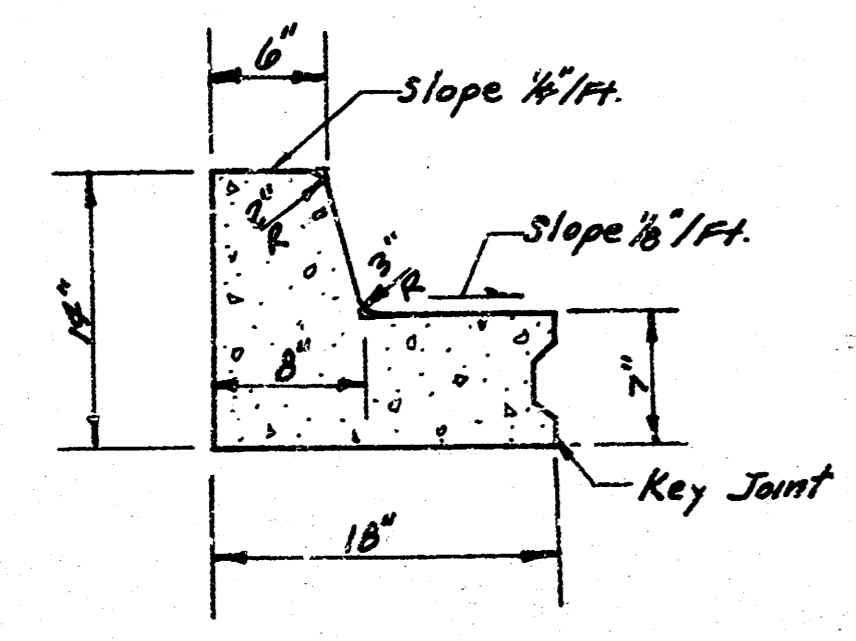
MEDIAL COMB. CURB & GTR.
