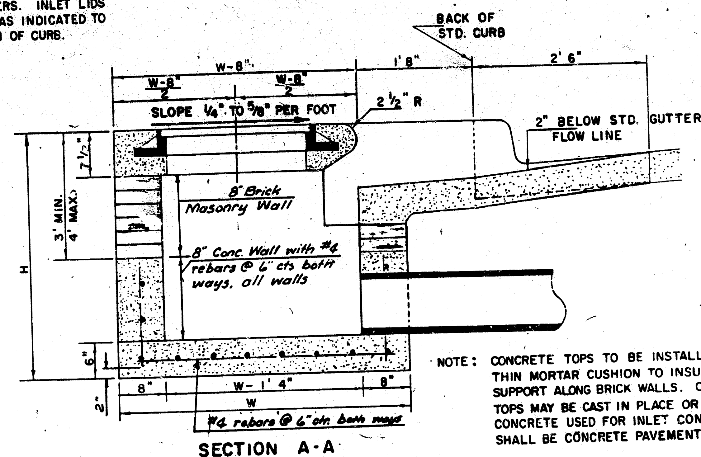
SECTION A-A
