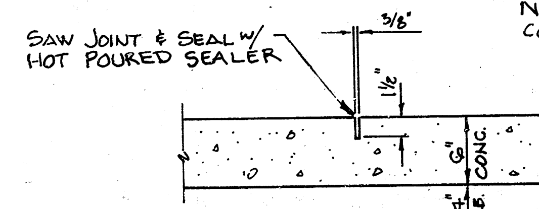
LONGITUDINAL JOINT
