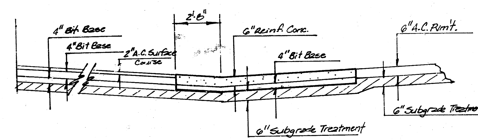
SECTION A-A
