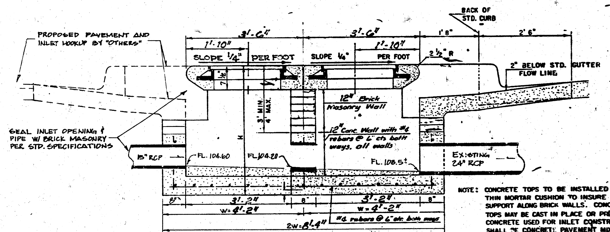
SECTION A-A
