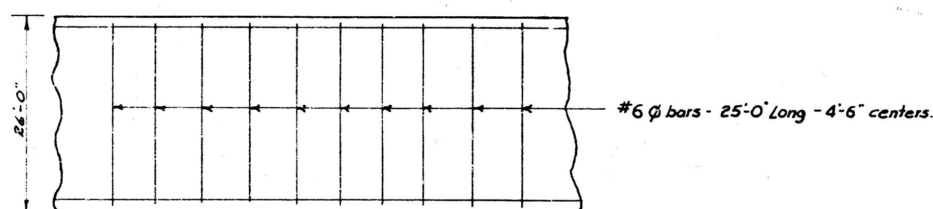
TYPICAL STEEL PATTERN Sta. 0+00 to Sta. 5+05.19 No Scale.
