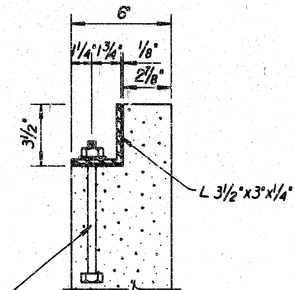
SECTION A-A
