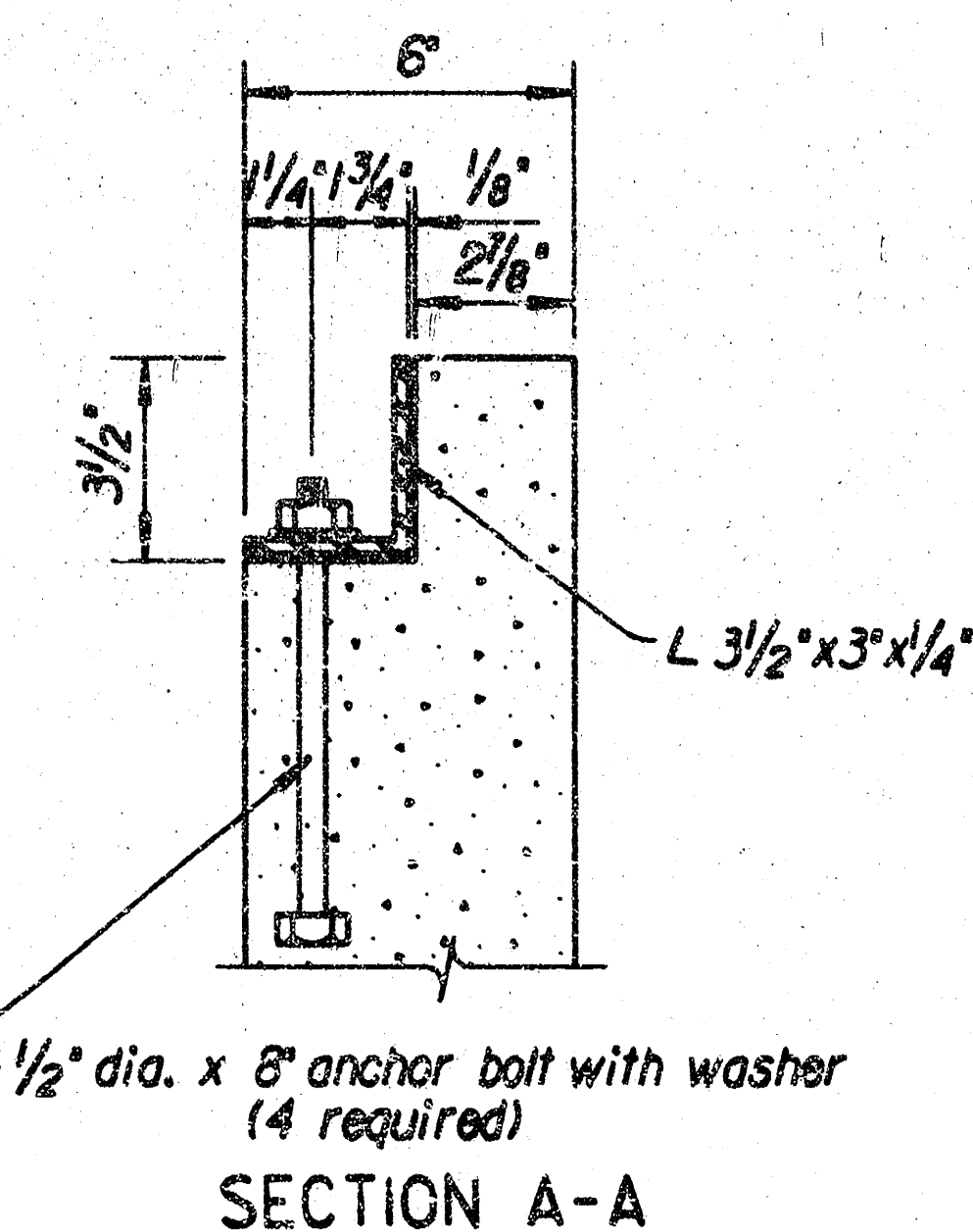
SECTION A-A
