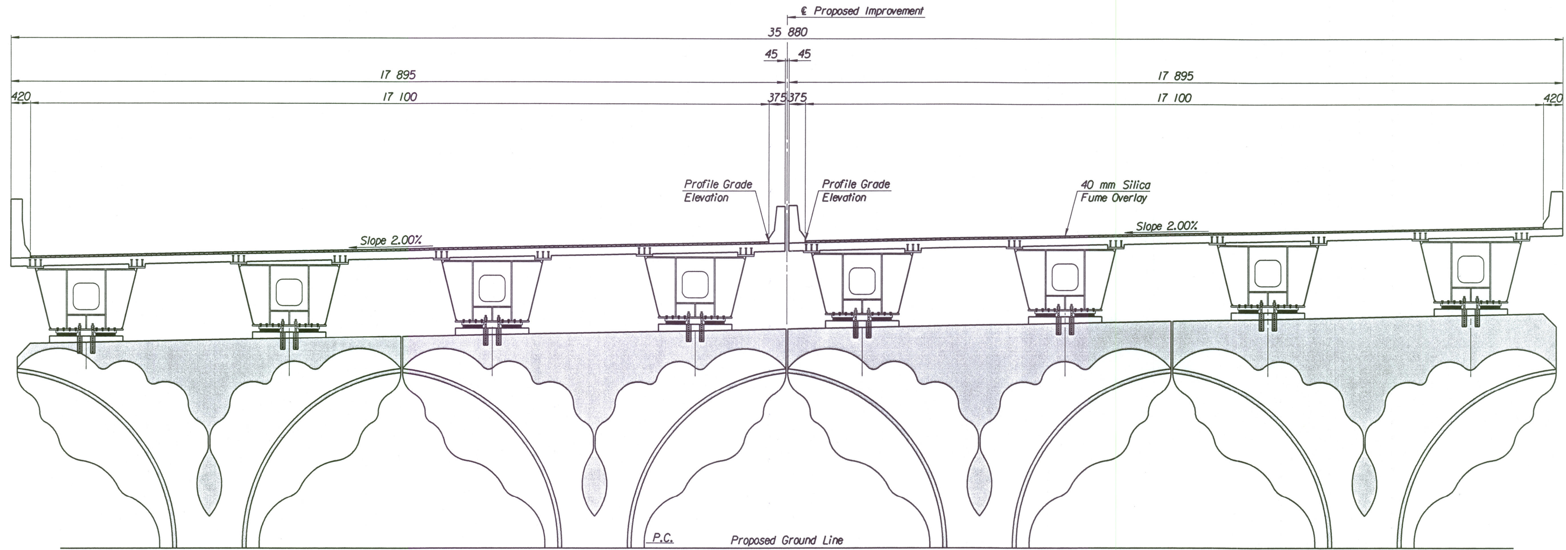
ELEVATION
