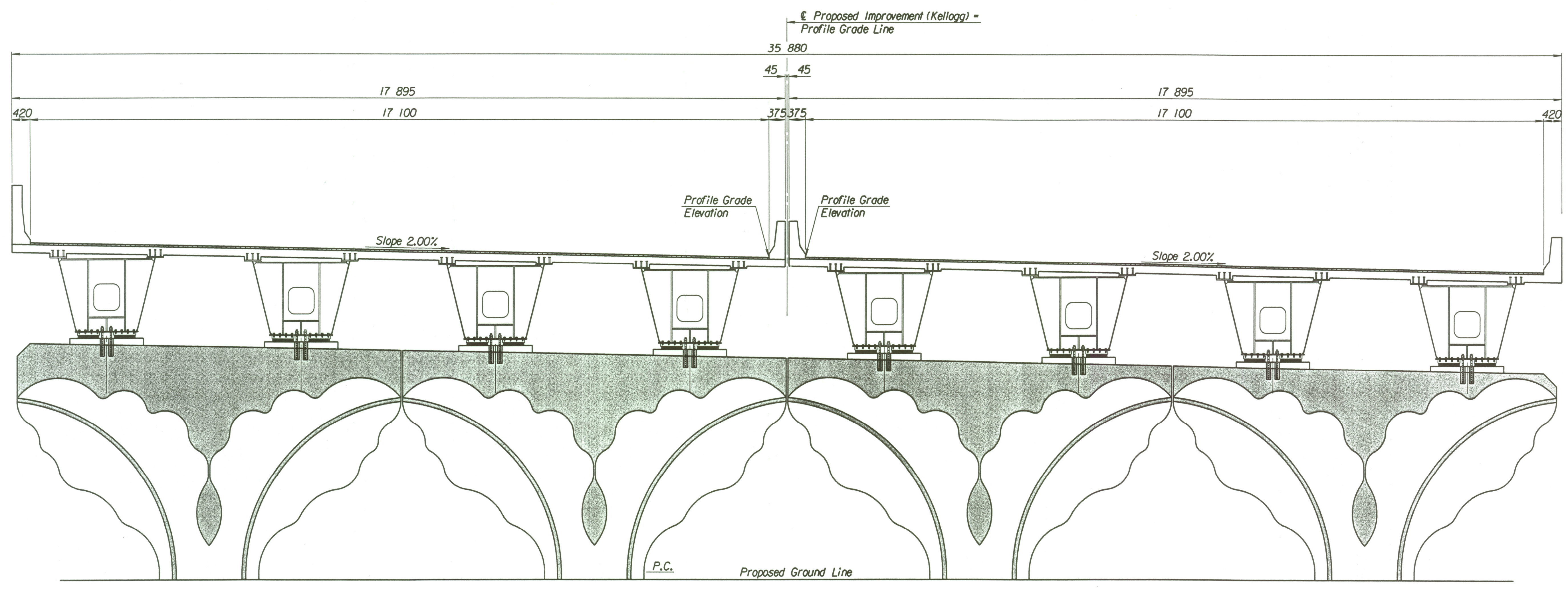
ELEVATION
