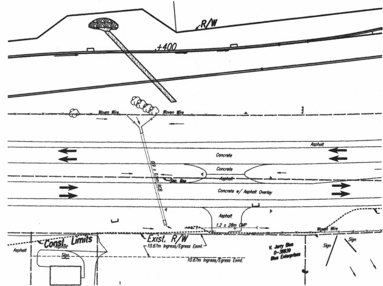
STA. 15+407 STAGE 1A ④
