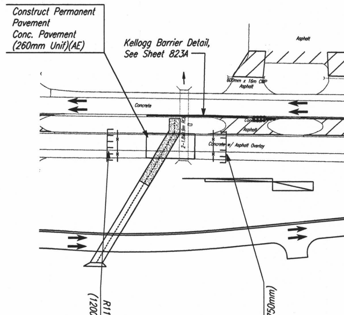
STA. 14+443 STAGE 3A ②
