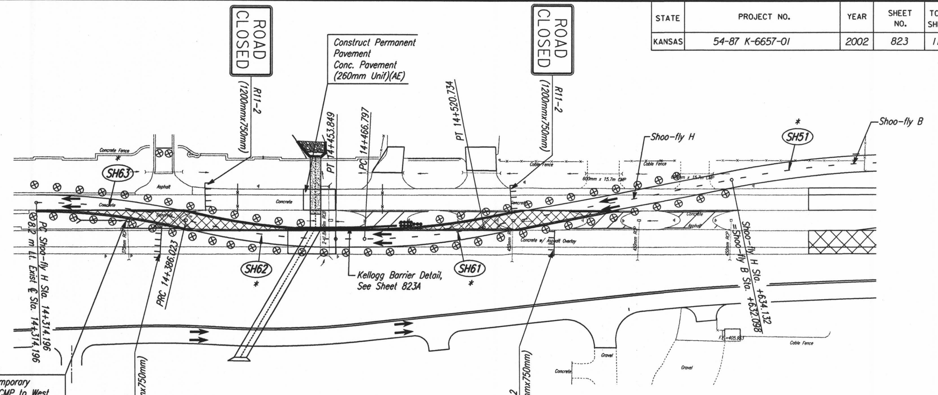
STA. 14+443 STAGE 3A ③
