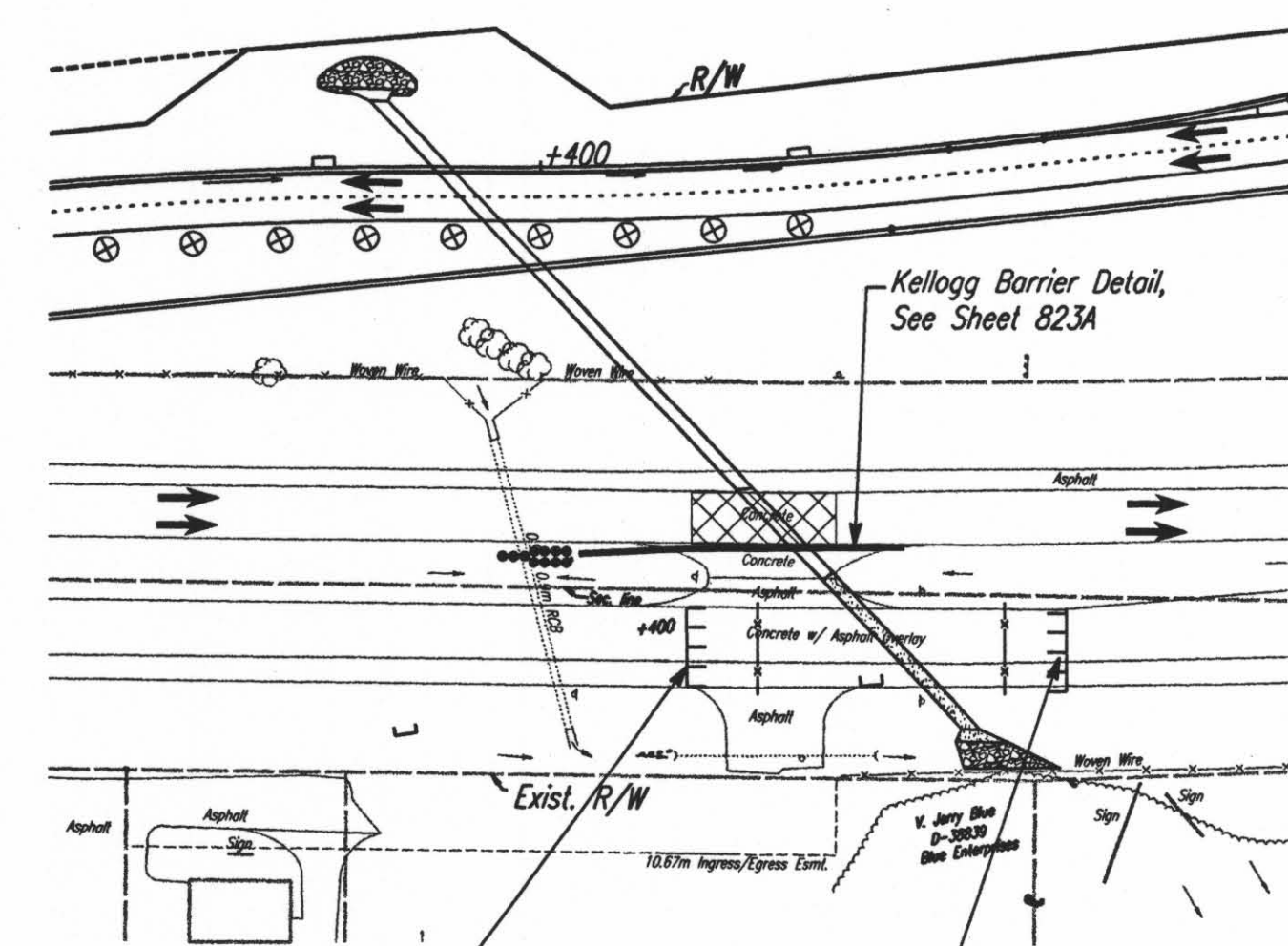
STA. 15+407 STAGE 2A ⑥
