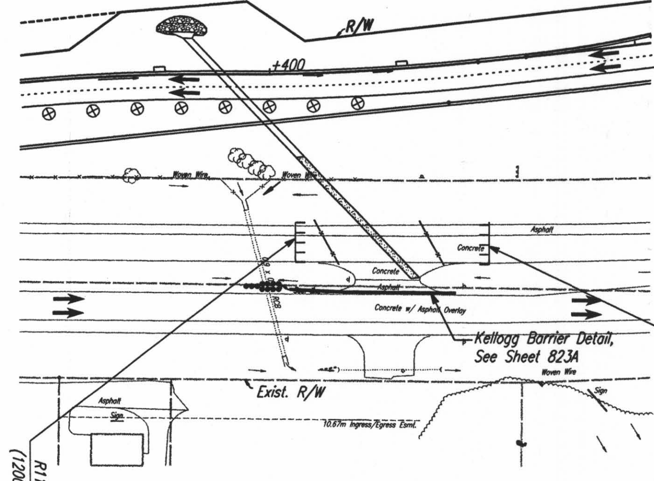
STA. 15+407 STAGE 2A ⑤
