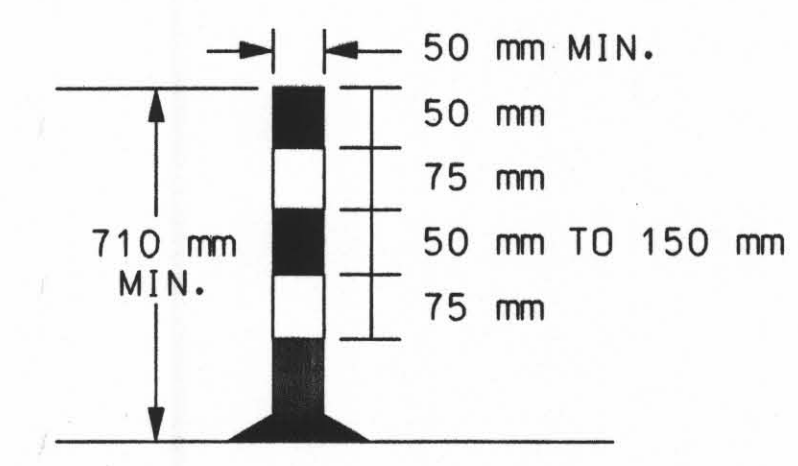
TUBULAR MARKERS
