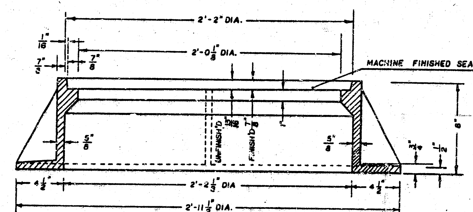
SECTION A-A
