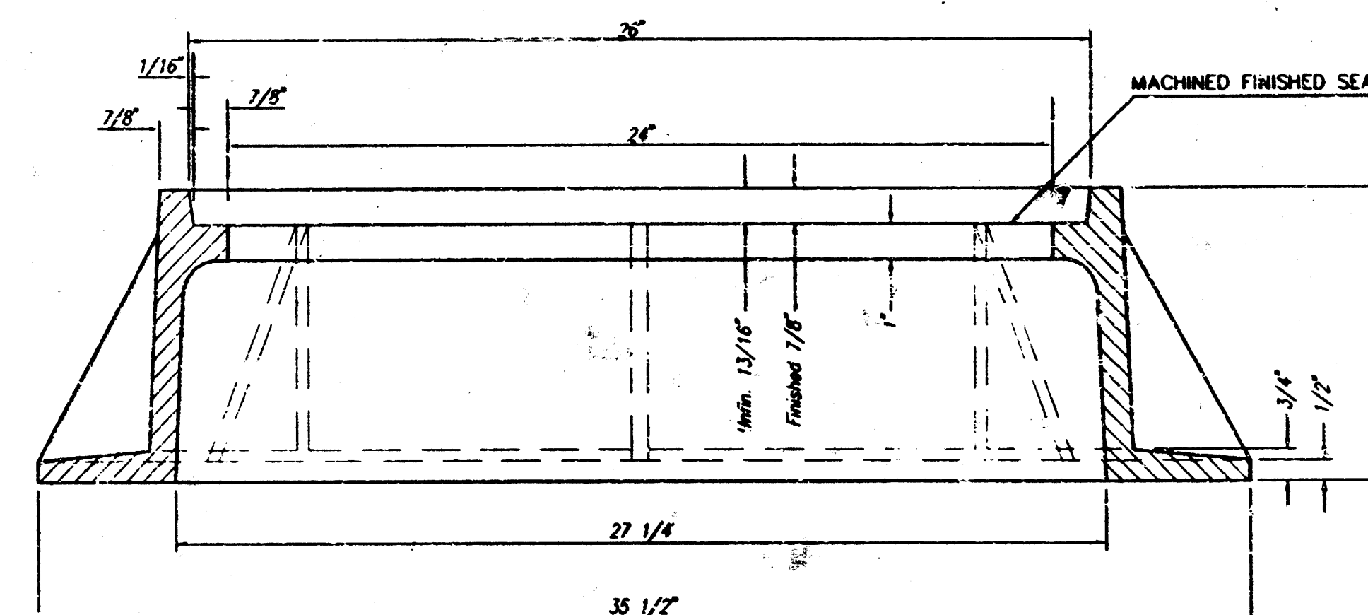
SECTION A-A
