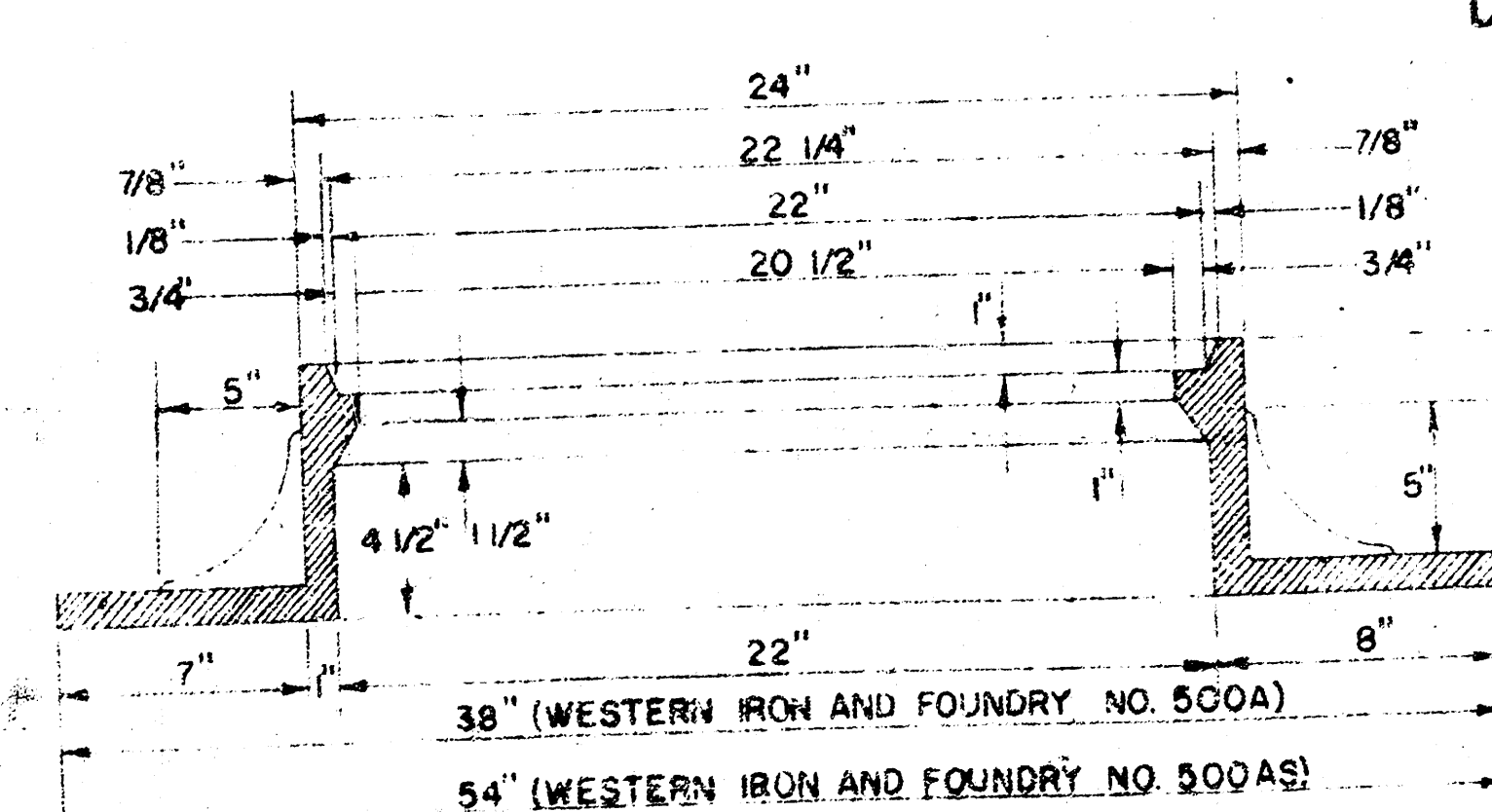
MANHOLE RING
