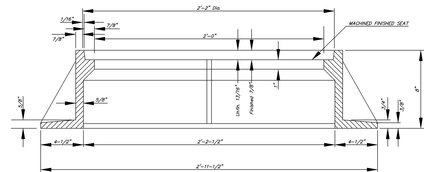
SECTION A-A
