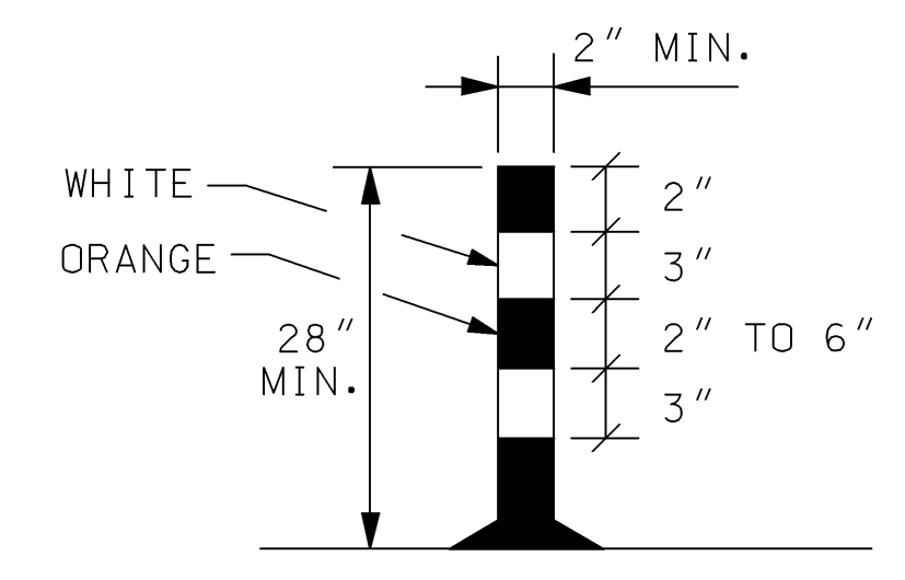
TUBULAR MARKER
