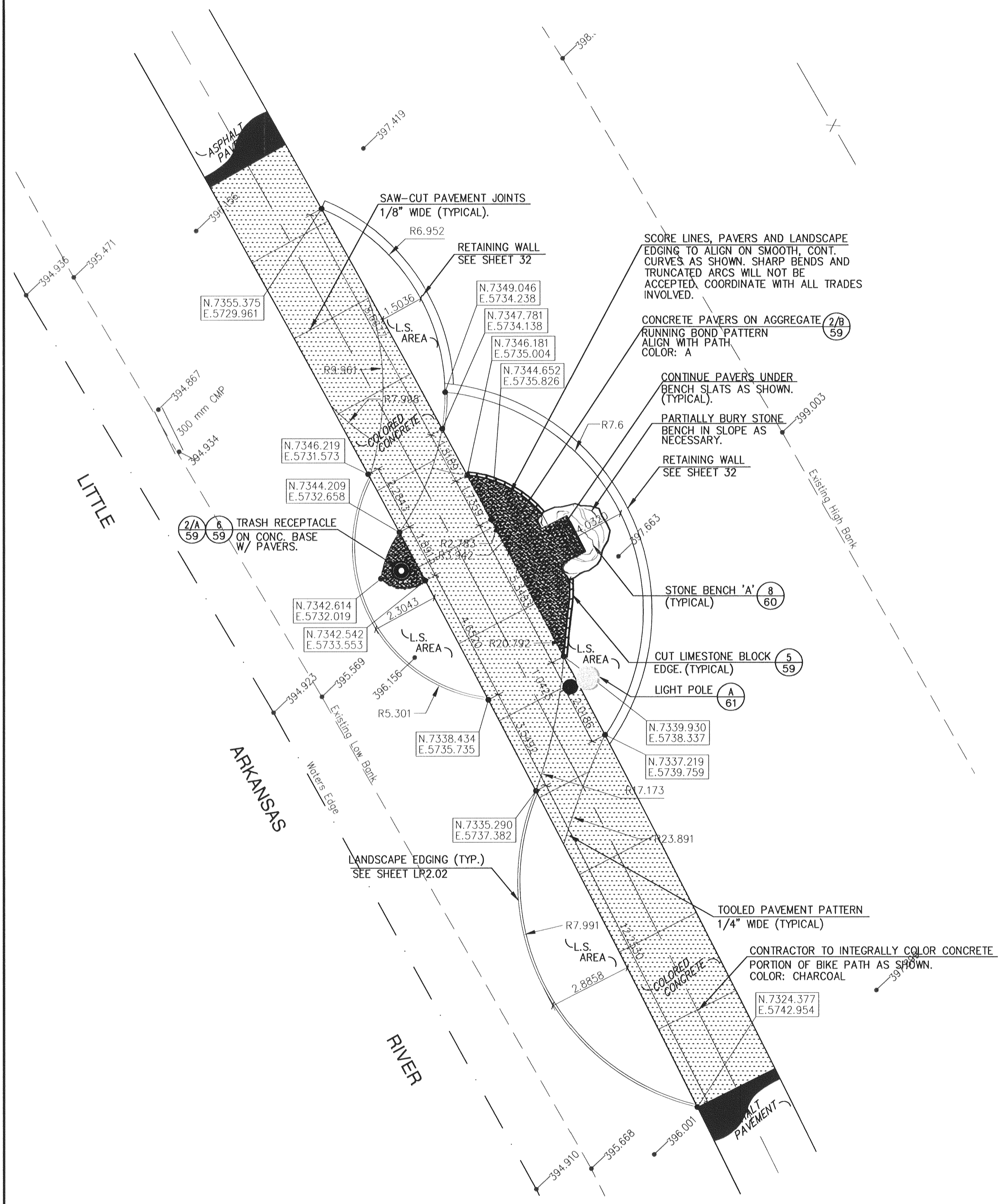
ENLARGED PAUSE POINT 'C' SCALE: 1:100
