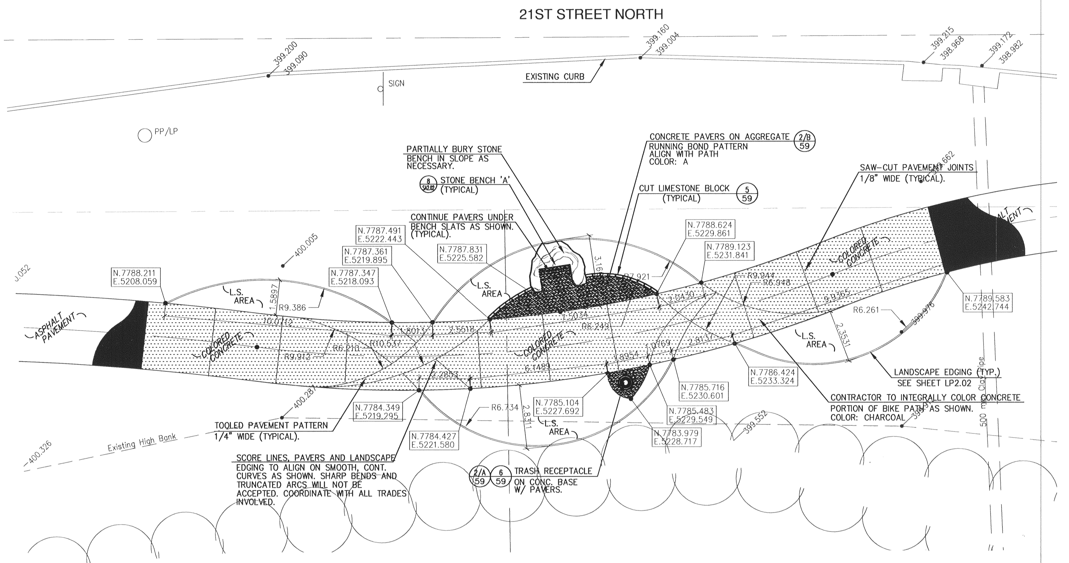
ENLARGED PAUSE POINT 'D' SCALE: 1:100
