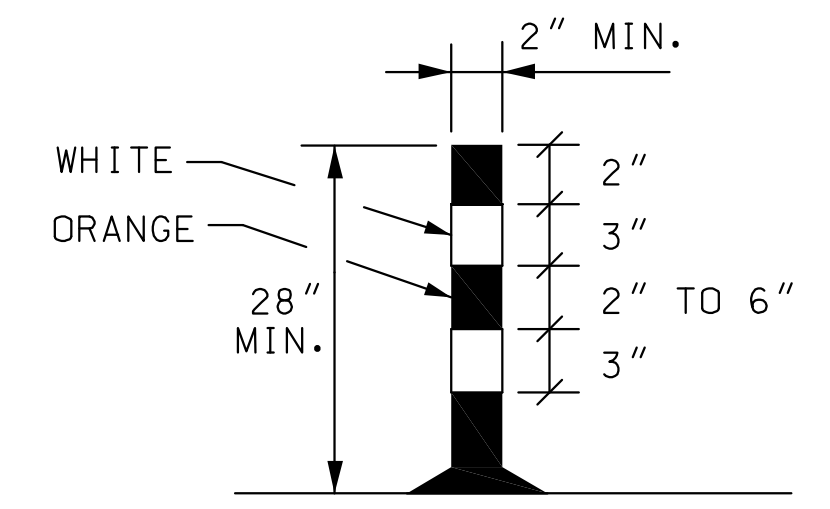
TUBULAR MARKER
