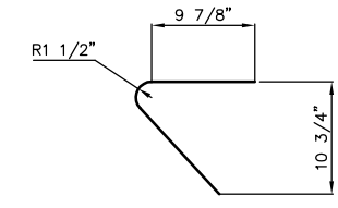
"A" Bar
