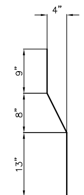
"B" Bar
