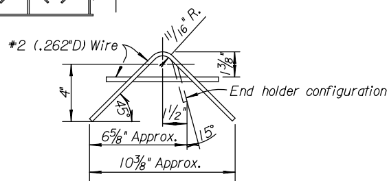
SEC. A-A
