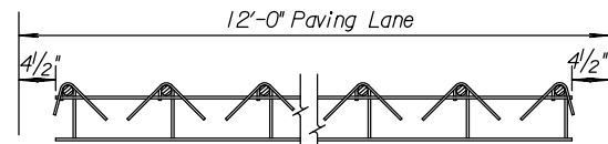
SEC. A-A
