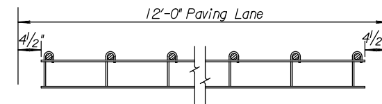
SEC. A-A
