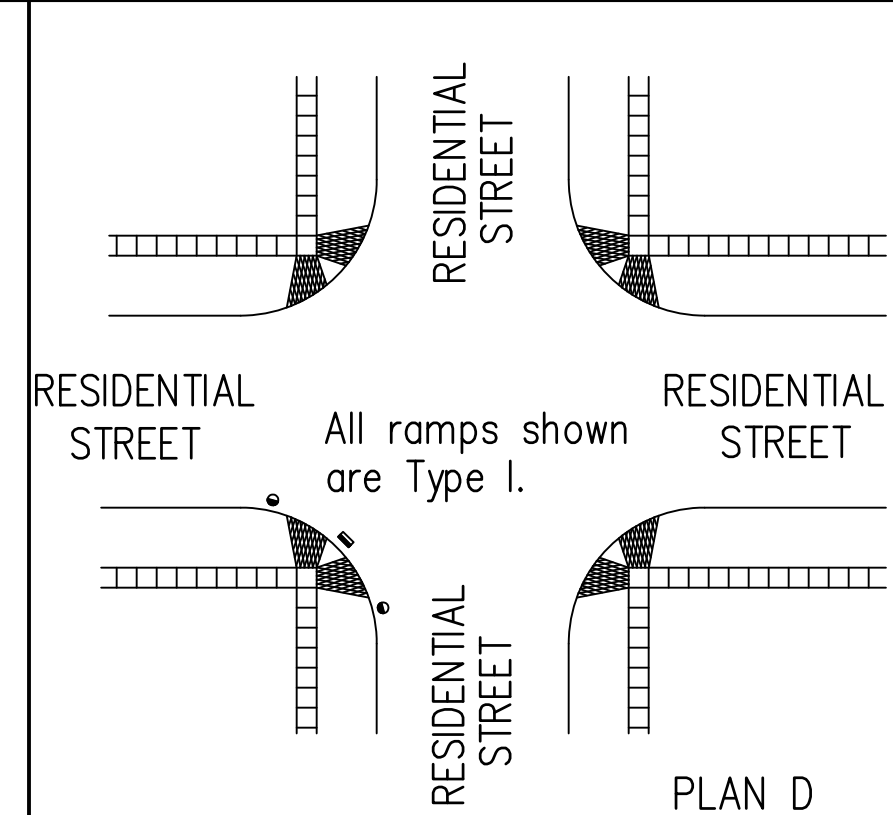
PLAN D
