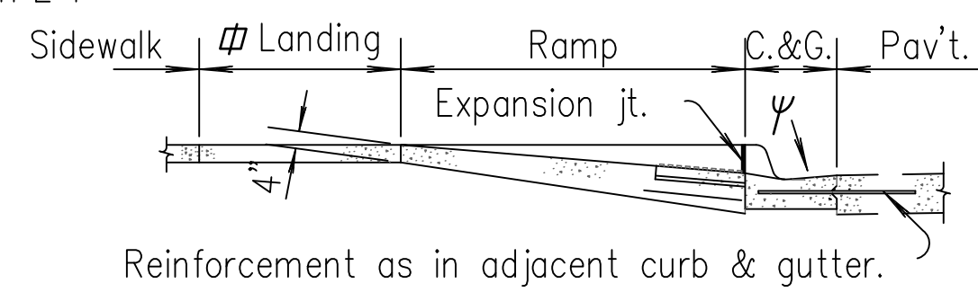
SECTION D-D
