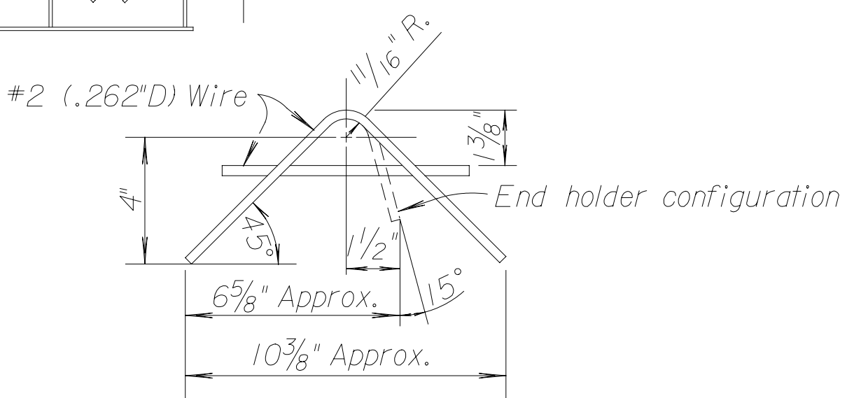
SEC. A-A
