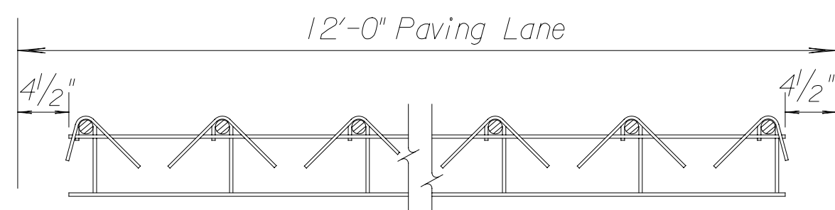
SEC. A-A
