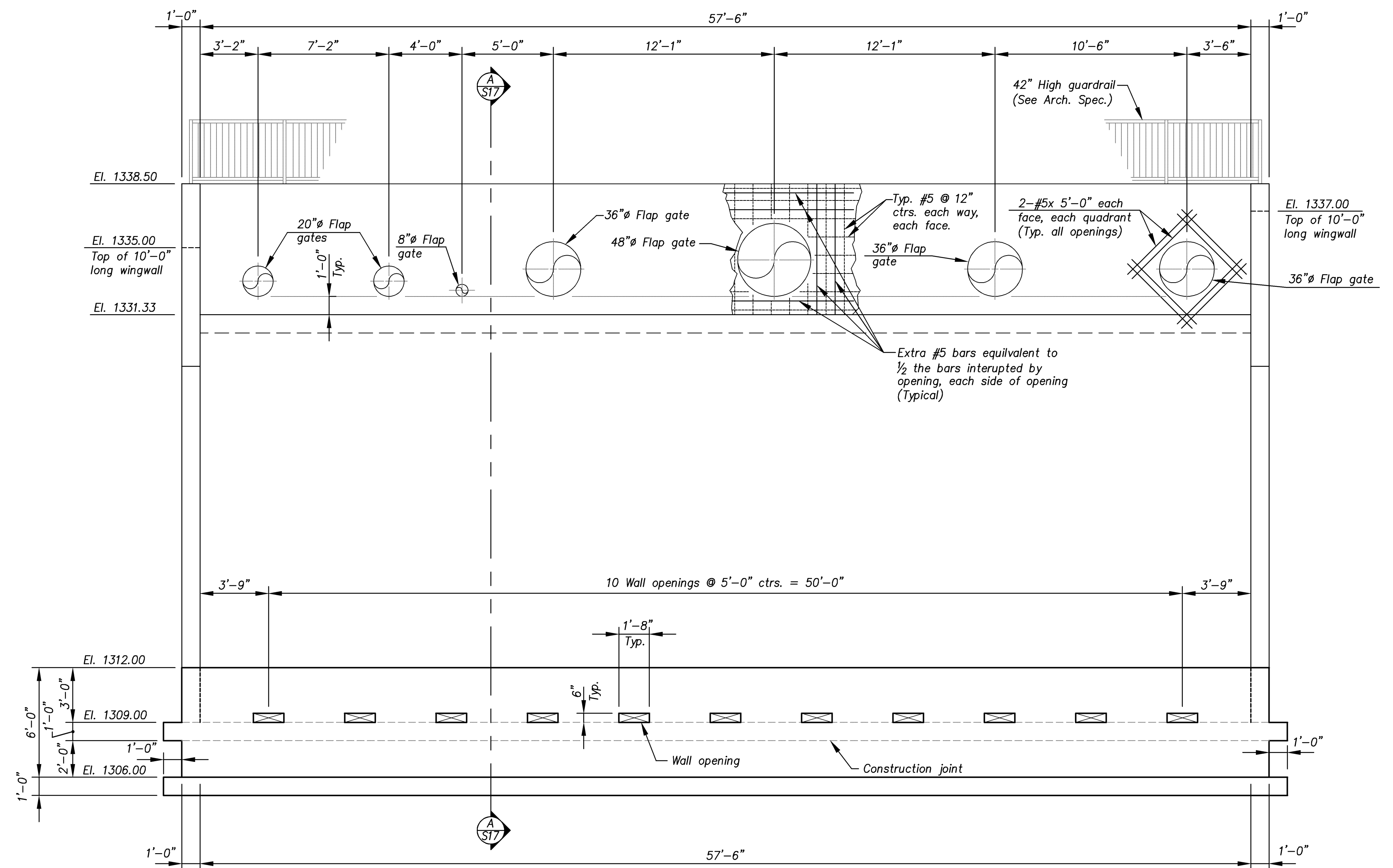
ELEVATION
