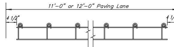
SEC. A-A
