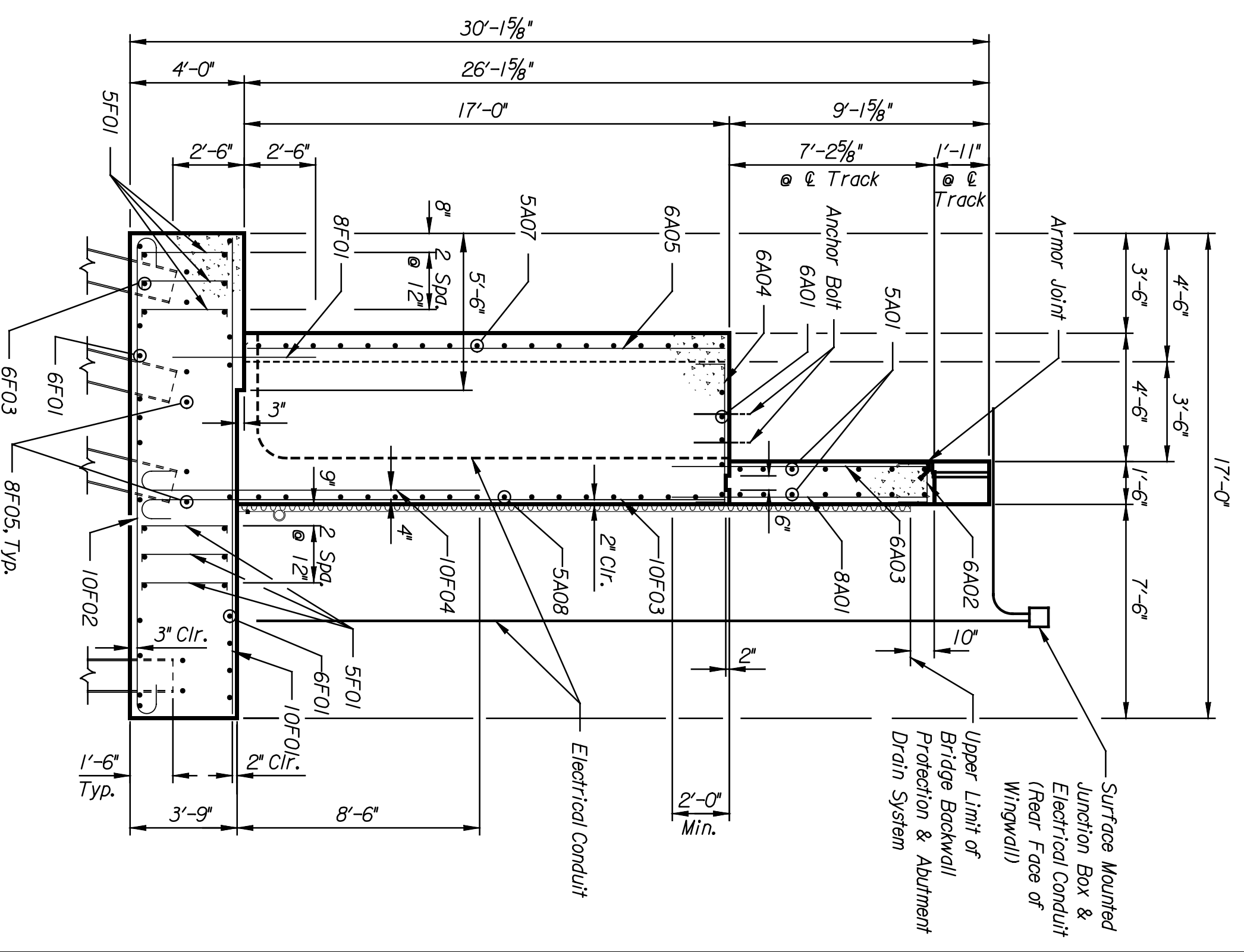
SECTION A Scale: 1/4" = 1'-0"
