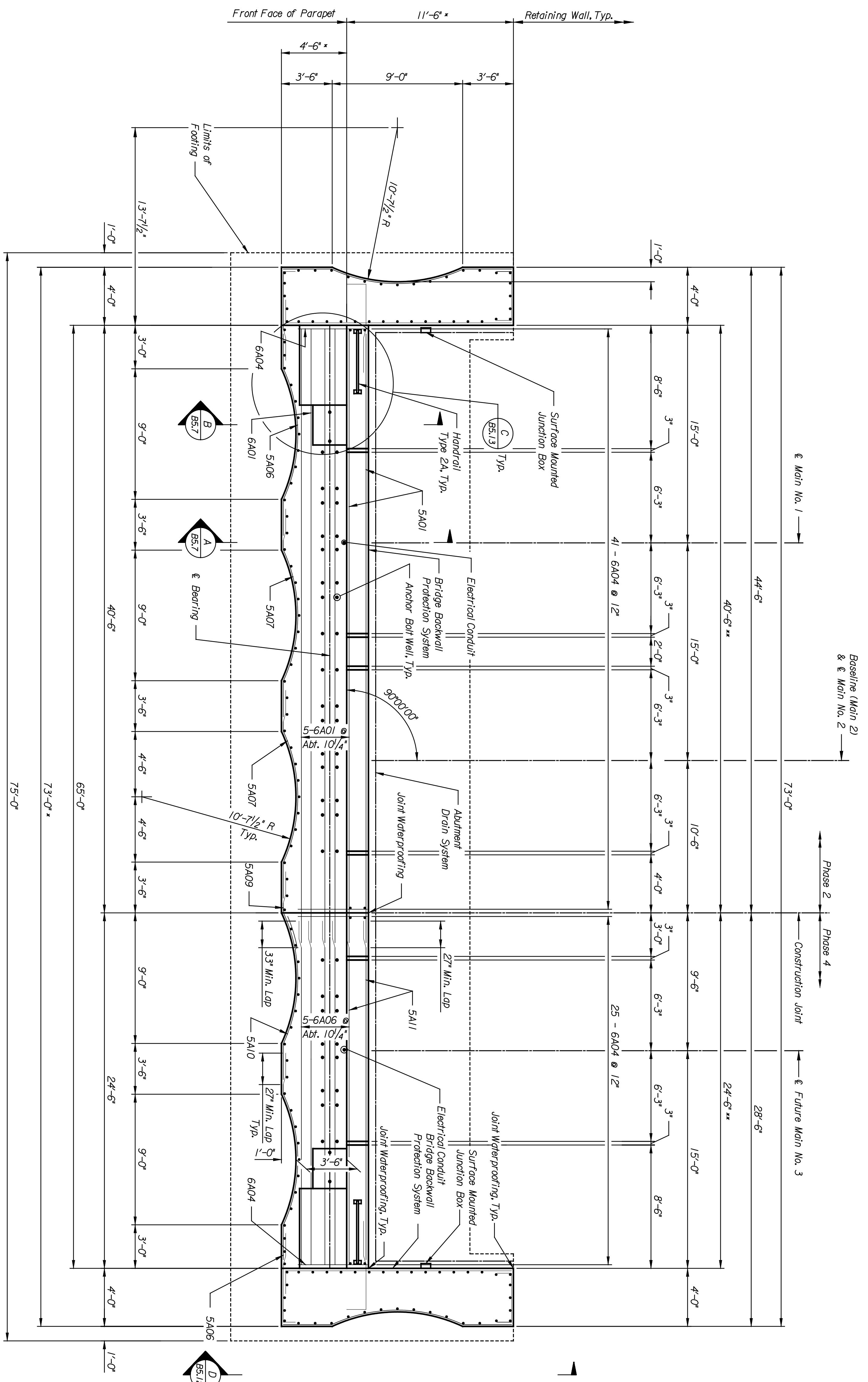
PLAN Scale: 1/4" = 1'-0"
