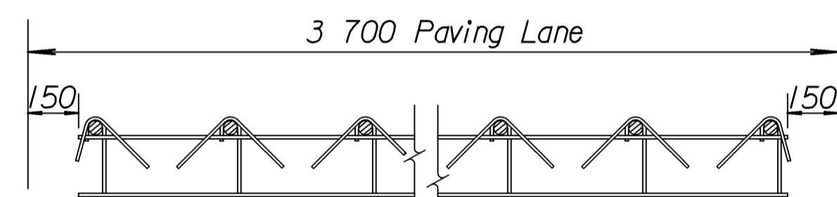
SEC. A-A
