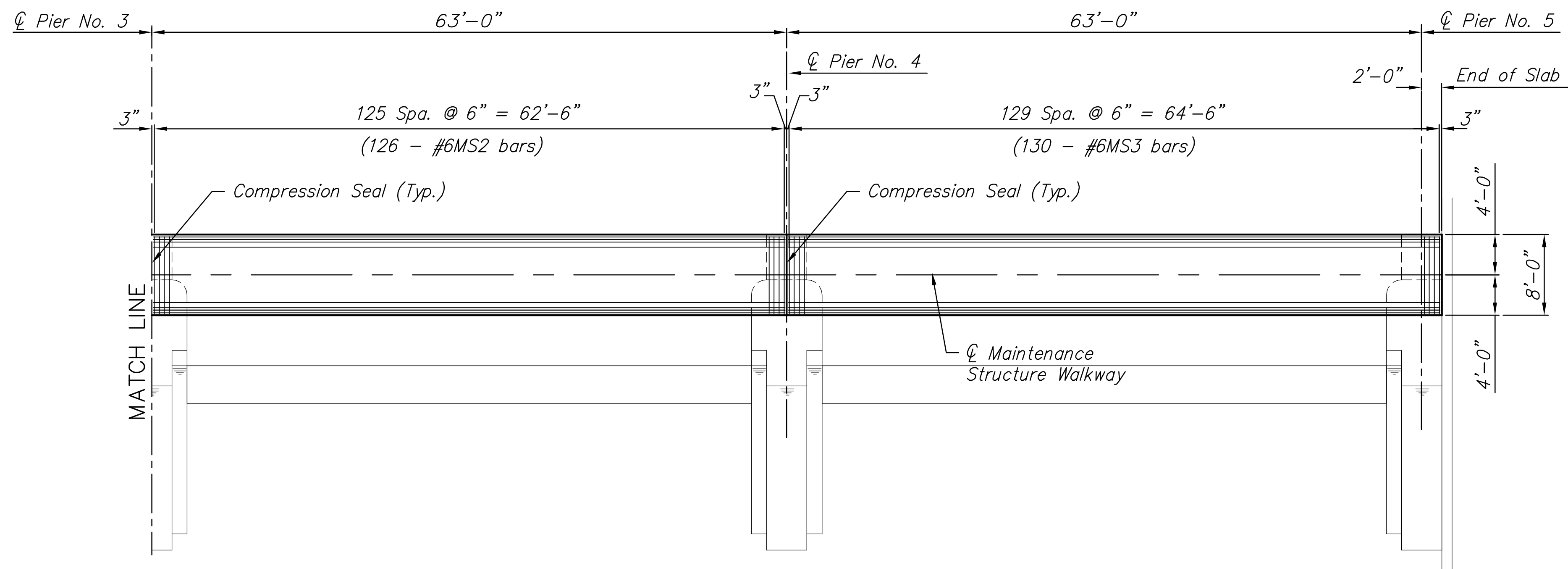
HALF PLAN SCALE: 1/8" = 1'-0"
