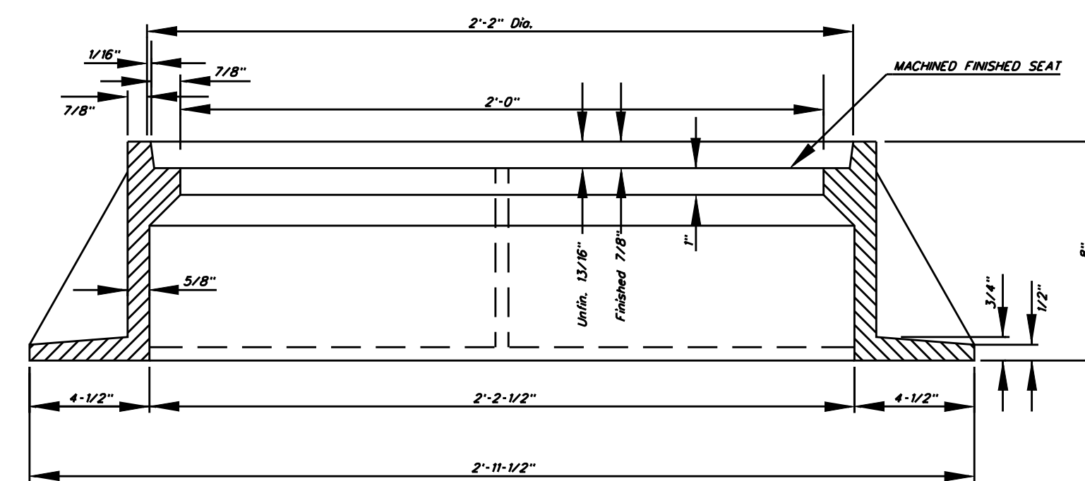
SECTION A-A
