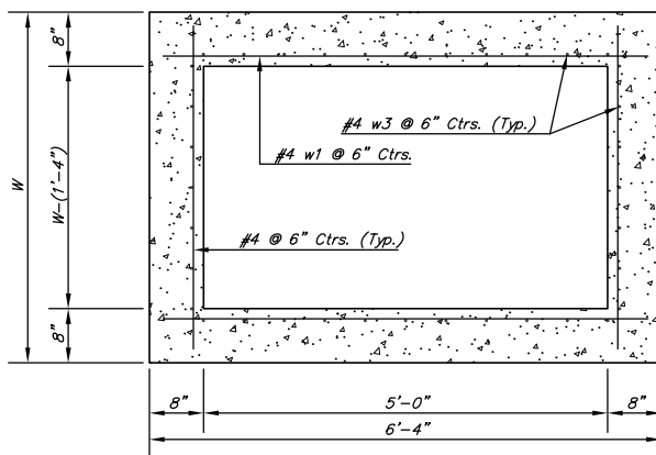
SECTION D-D
