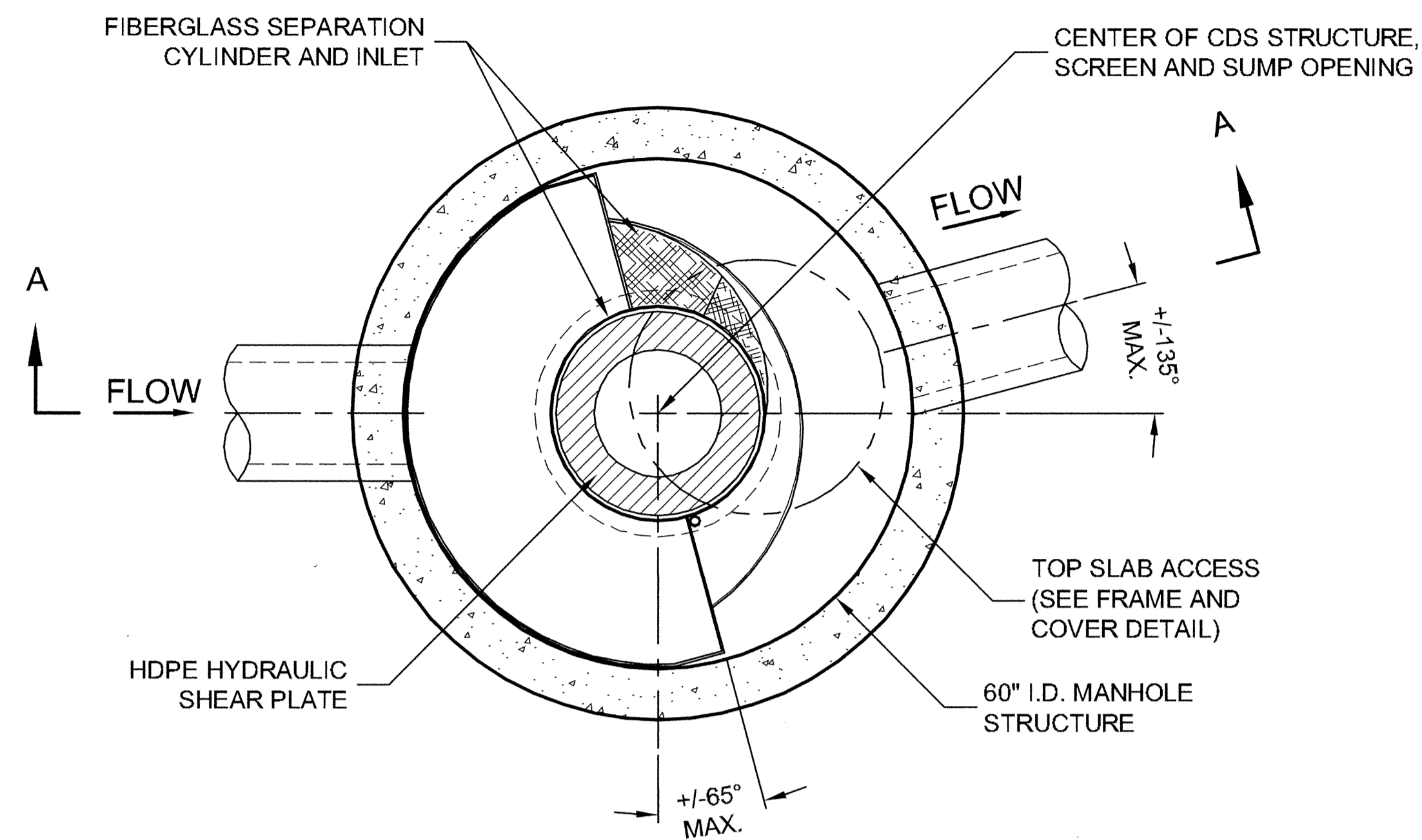
PLAN VIEW B-B N.T.S.
