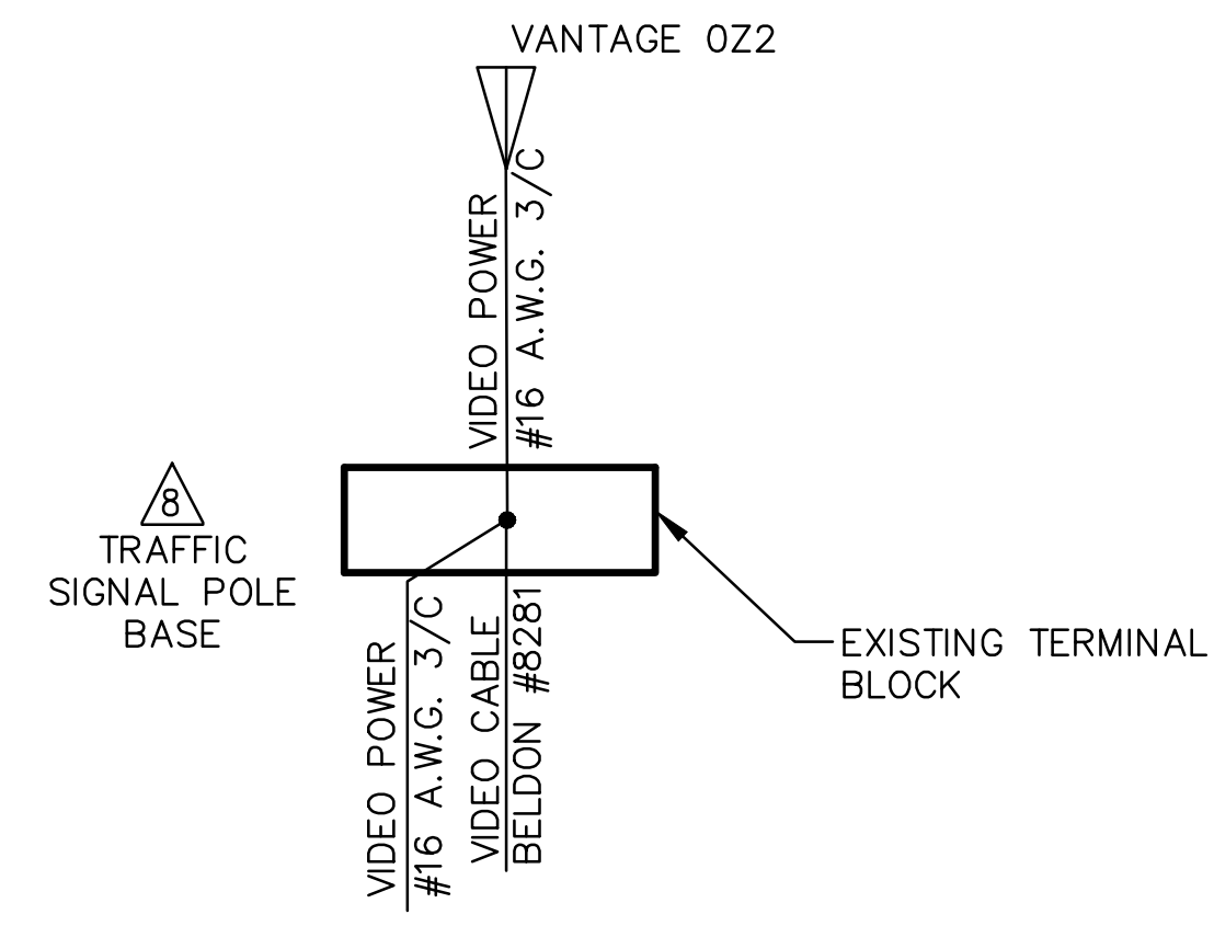
POLE WIRING DIAGRAMS
