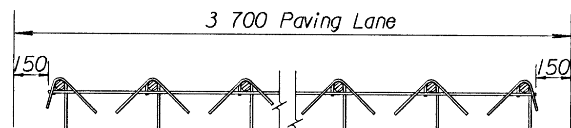
SEC. A-A
