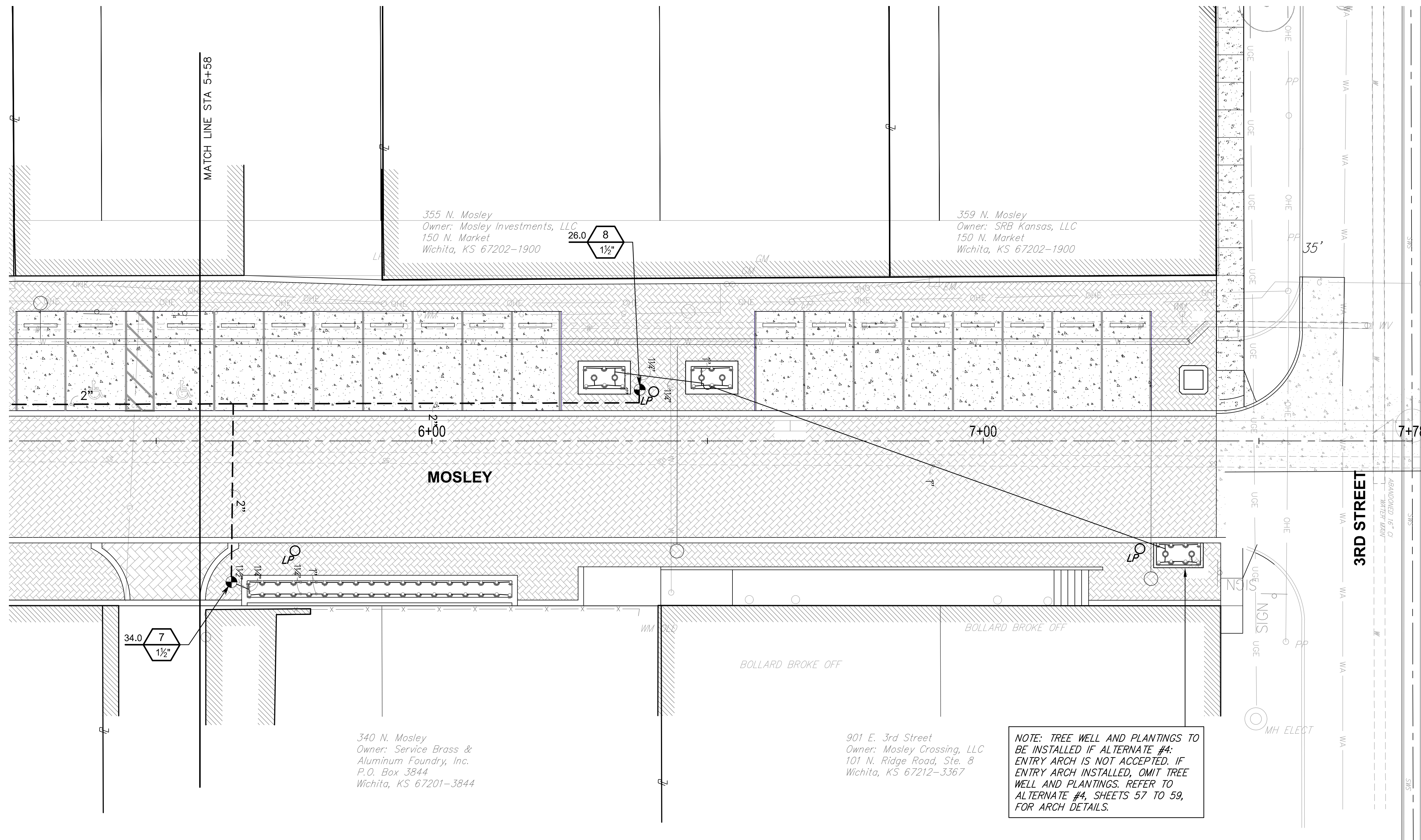
IRRIGATION PLAN - STA 5+58 TO STA 7+78 SCALE: 1" = 10'
