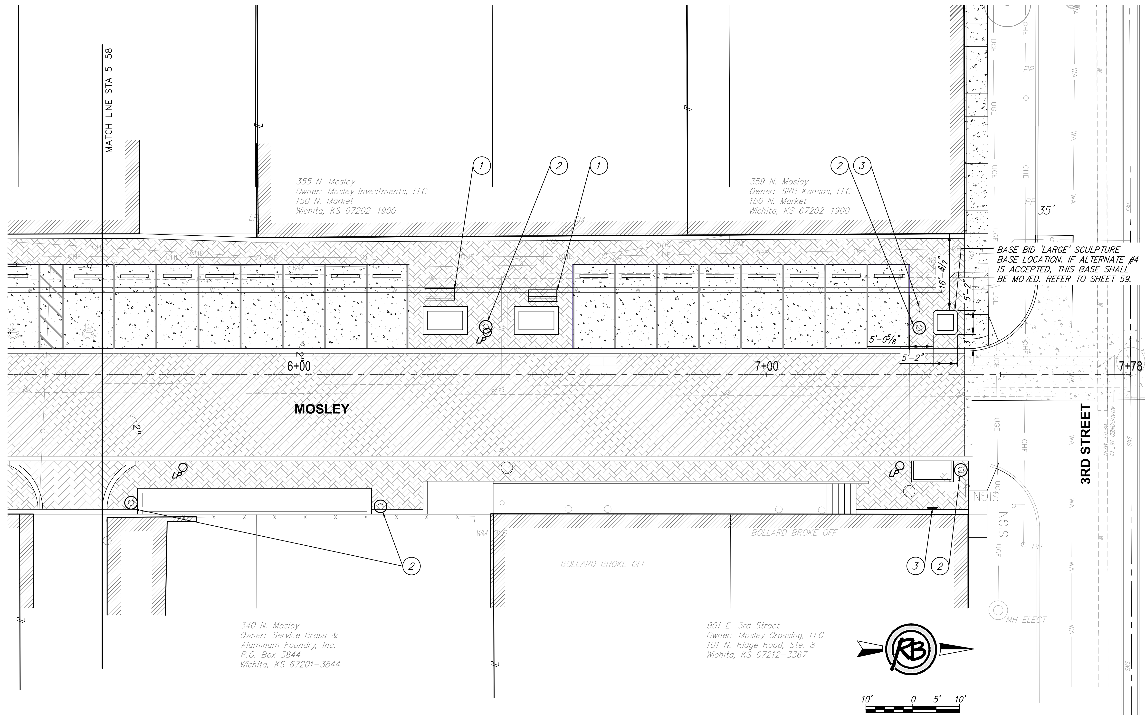
FURNISHINGS PLAN - STA 5+58 TO STA 7+78 SCALE: 1" = 10'
