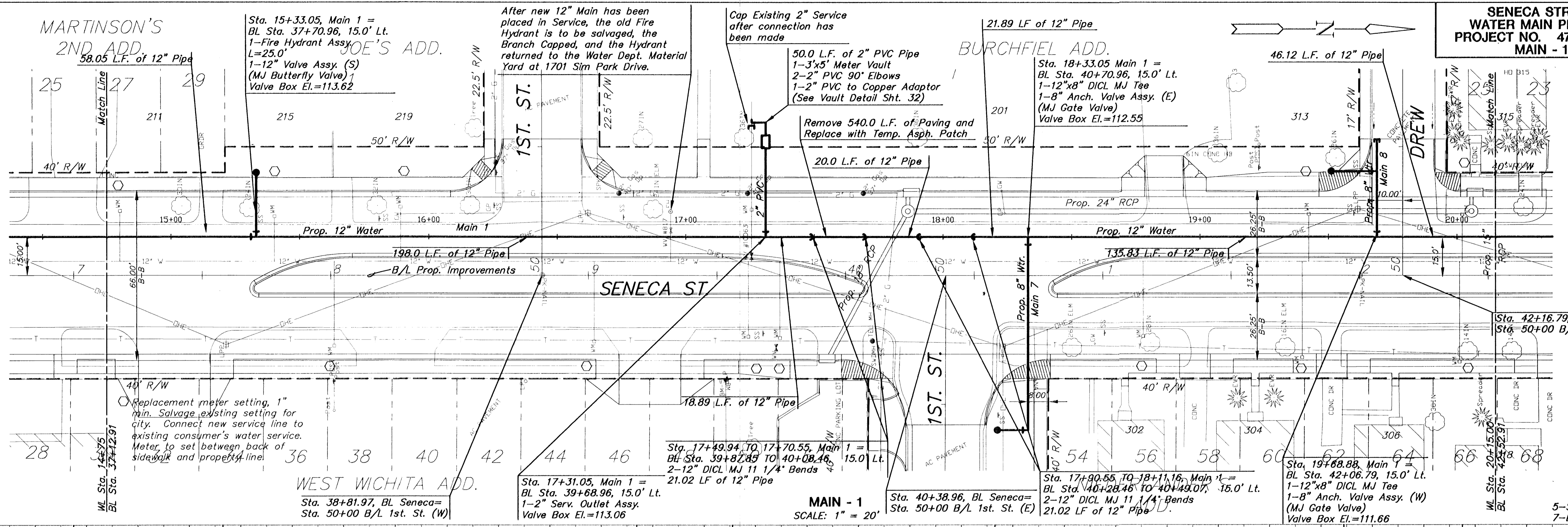
PROFILE - MAIN 1 HORIZONTAL SCALE: 1" = 20' VERTICAL SCALE: 1" = 5'
