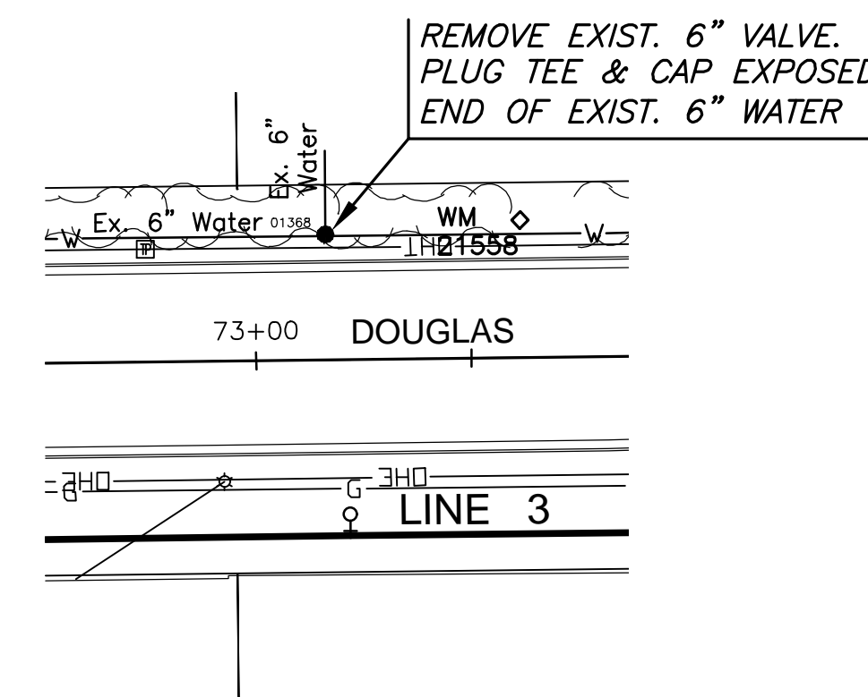
DOUGLAS STA. 73+00 DISCONNECT #23
