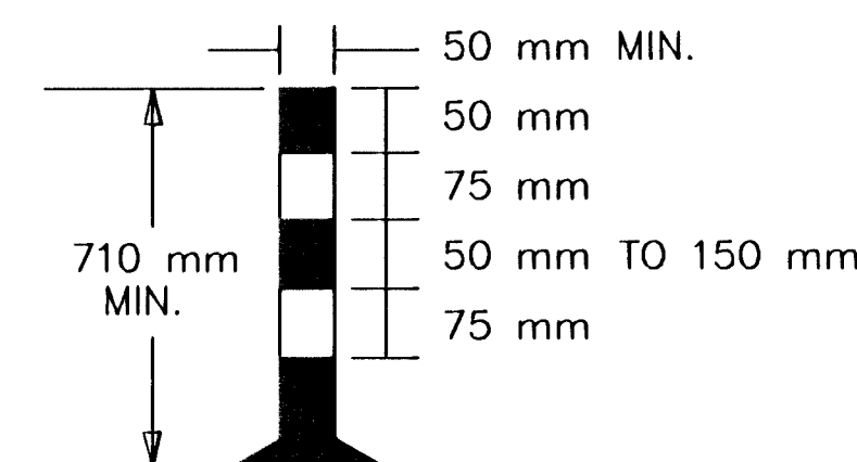
TUBULAR MARKERS
