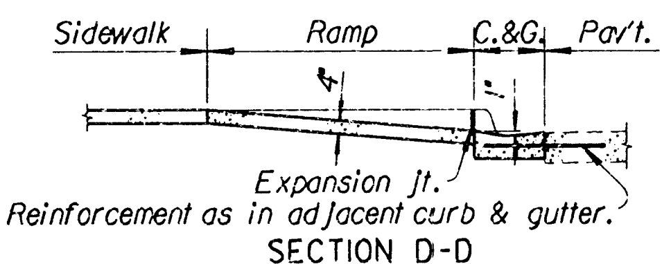
SECTION D-D
