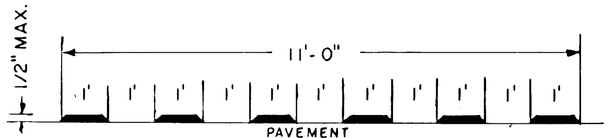
Section A-A
