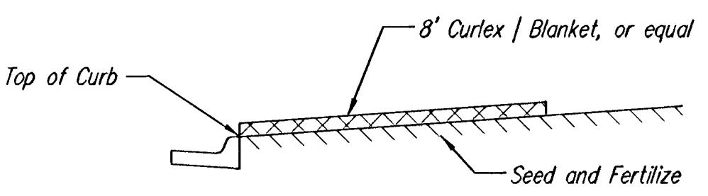
SECTION A-A
