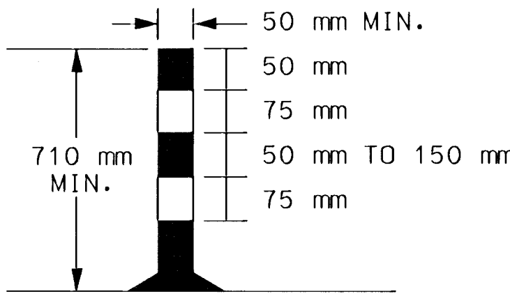
TUBULAR MARKERS
