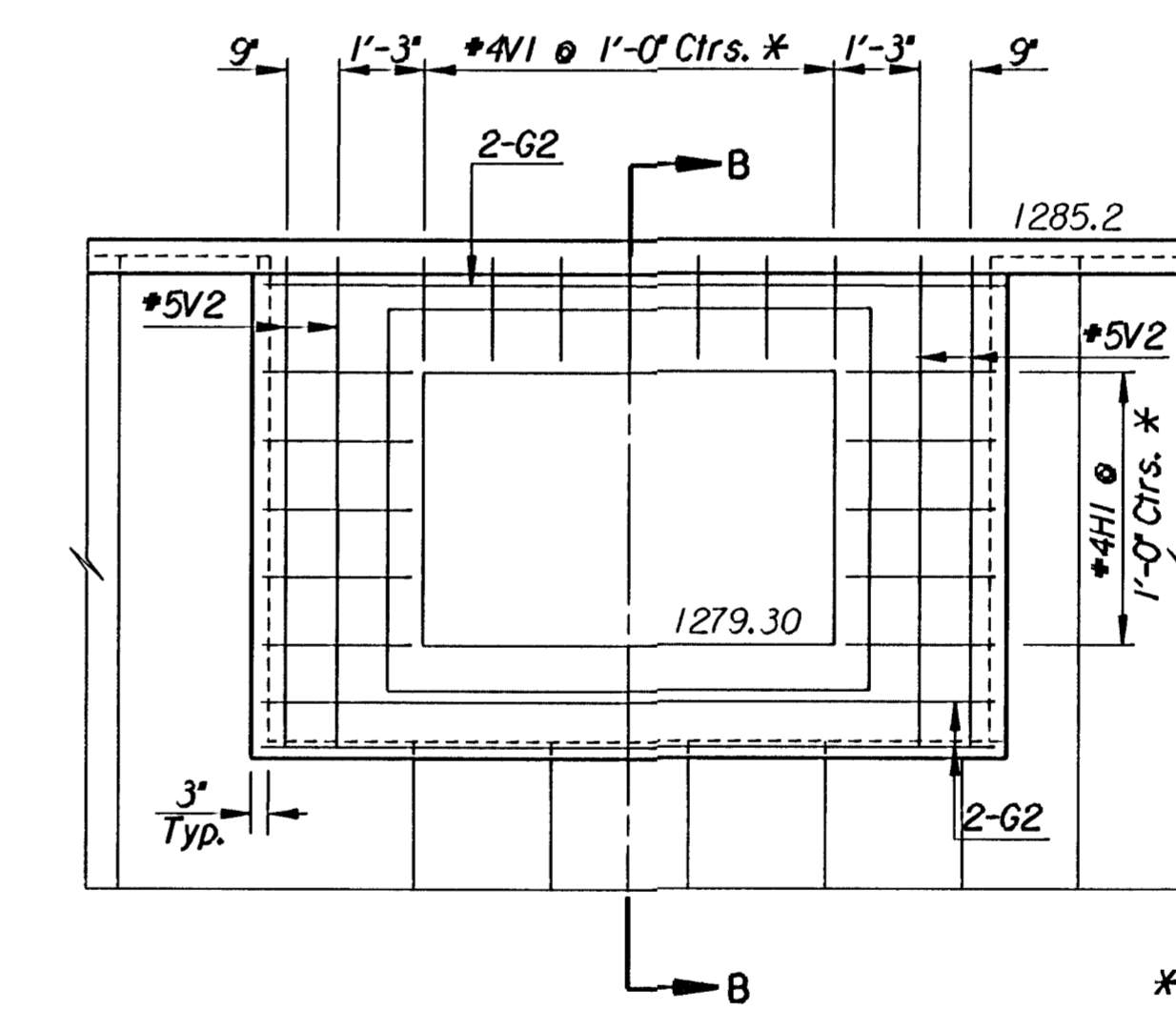
ELEVATION
