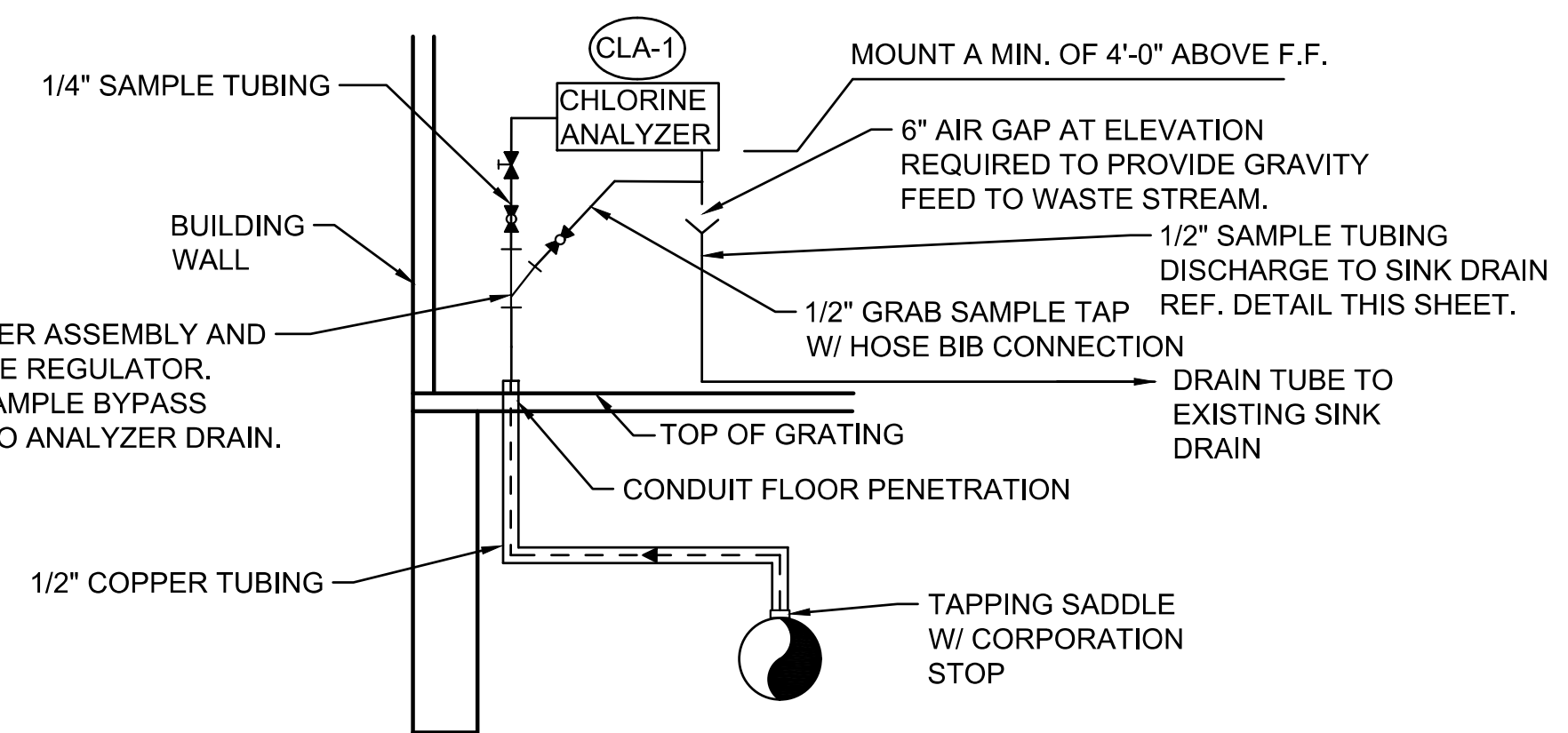
CHLORINE ANALYZER SCHEMATIC SCALE: N.T.S.
