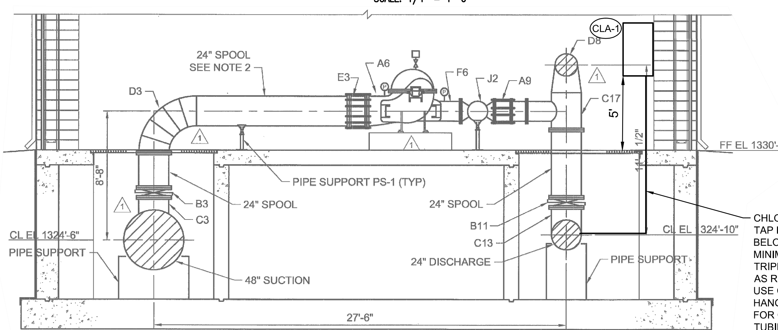
1 SECTION SCALE: 1/4" = 1'-0"
