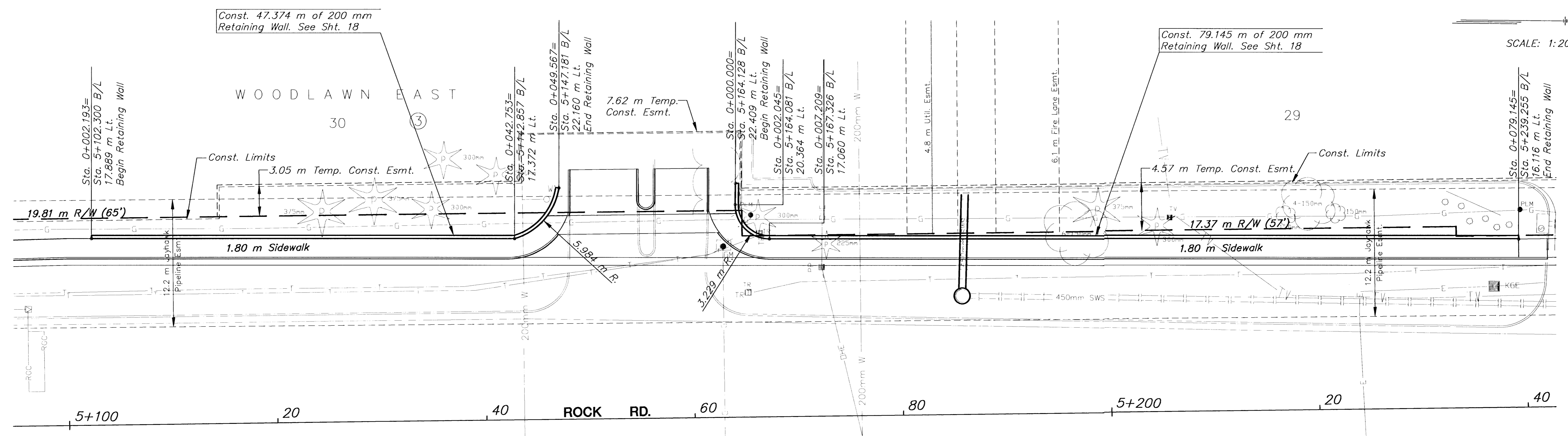
PLAN - WALL 1 & WALL 2 Scale: 1:200
