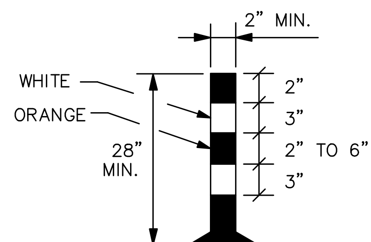
TUBULAR MARKER
