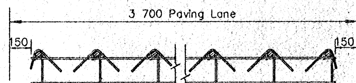
SEC. A-A
