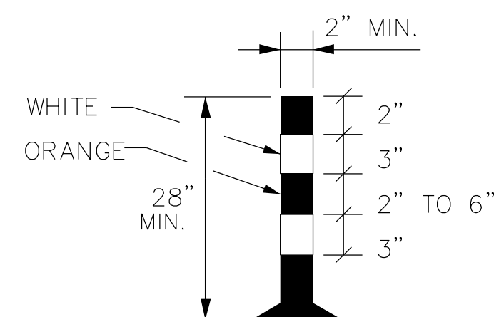
TUBULAR MARKER
